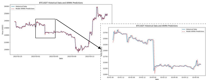
рис. – Результат комп'ютерної програми за моделлю ARIMA
