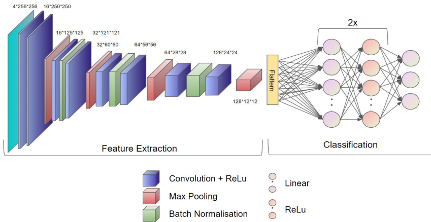
Мал. 1. Архітектура моделі
