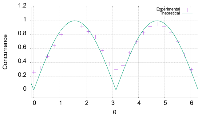
Рис. 1: Експериментальні результати обчислення узгодженості стану |\chi(\theta)\rangle (6) для різних значень параметра \theta за формулою (3) на квантовому комп'ютері IBM Lima (+) та теоретичні (неперервна лінія).
