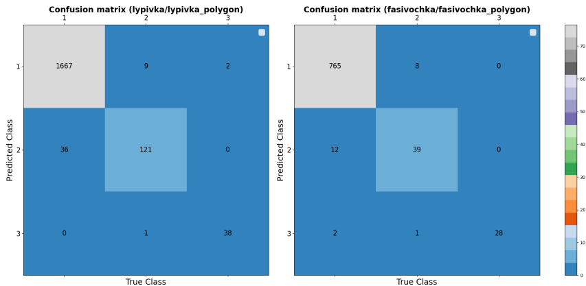
Мал. 2. Матриці конфузій
